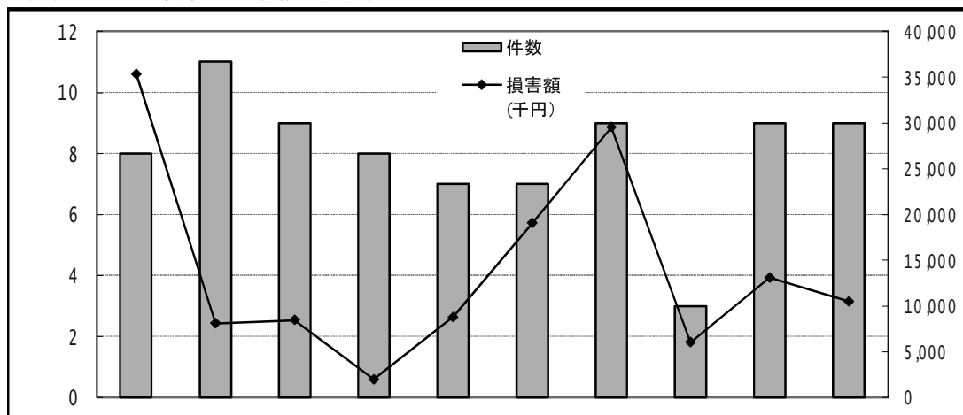
(1) 過去10年間の火災件数と損害額
