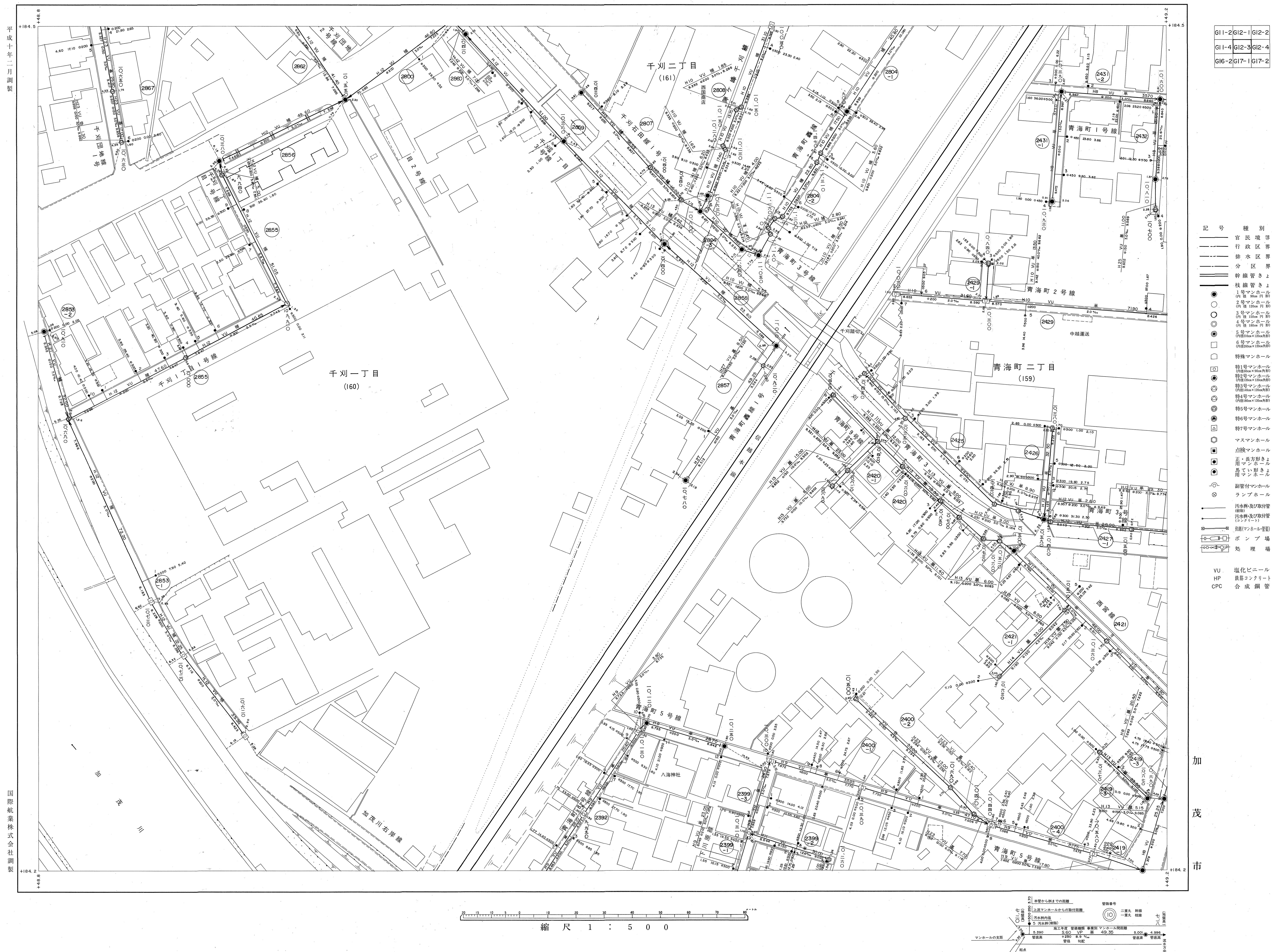
加茂市公共下水道台帳施設平面図 G12-3 (汚水)
