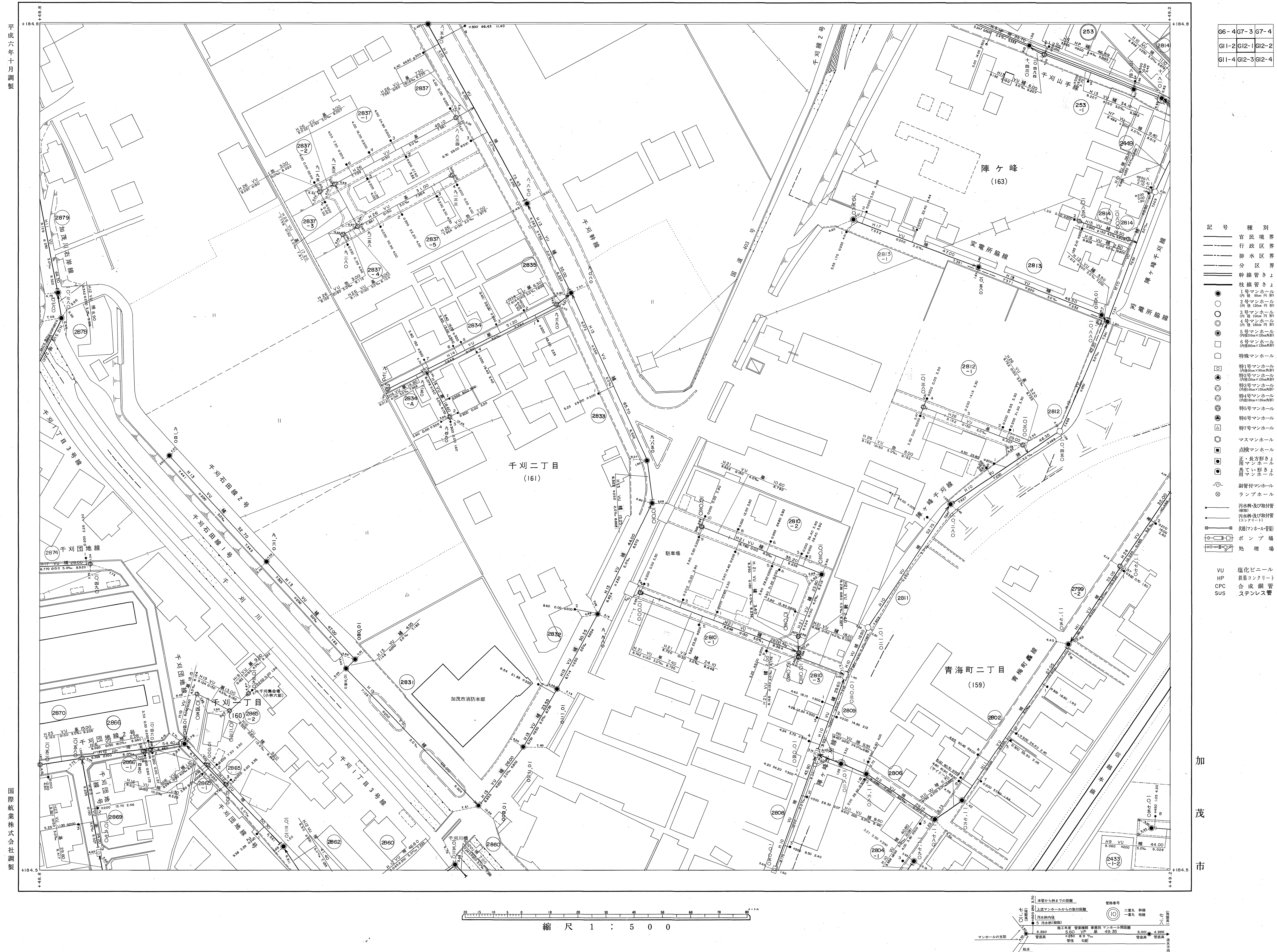
加茂市公共下水道台帳施設平面図 G12-1 (汚水)
