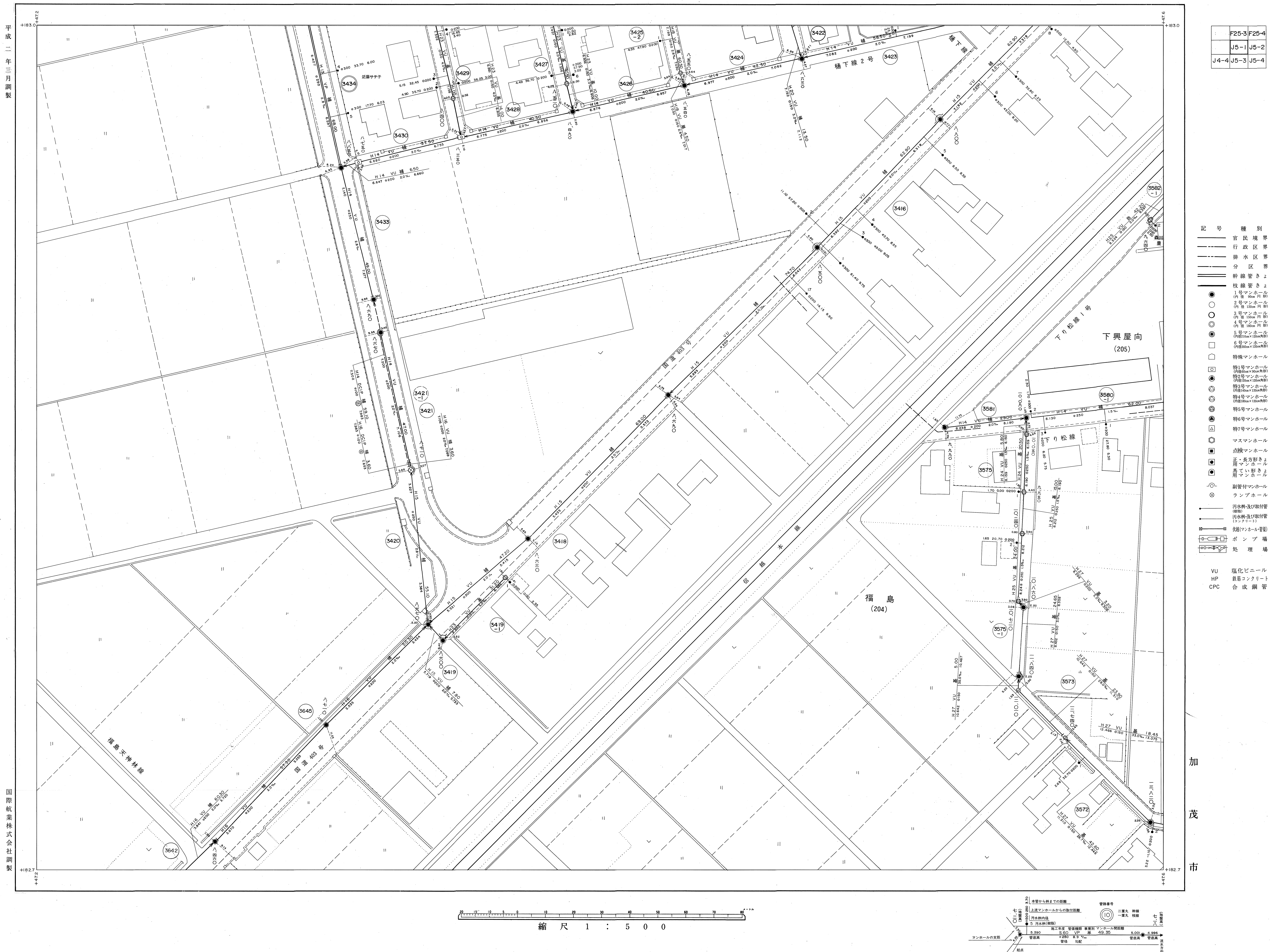
加茂市公共下水道台帳施設平面図 J5-1 (汚水)
