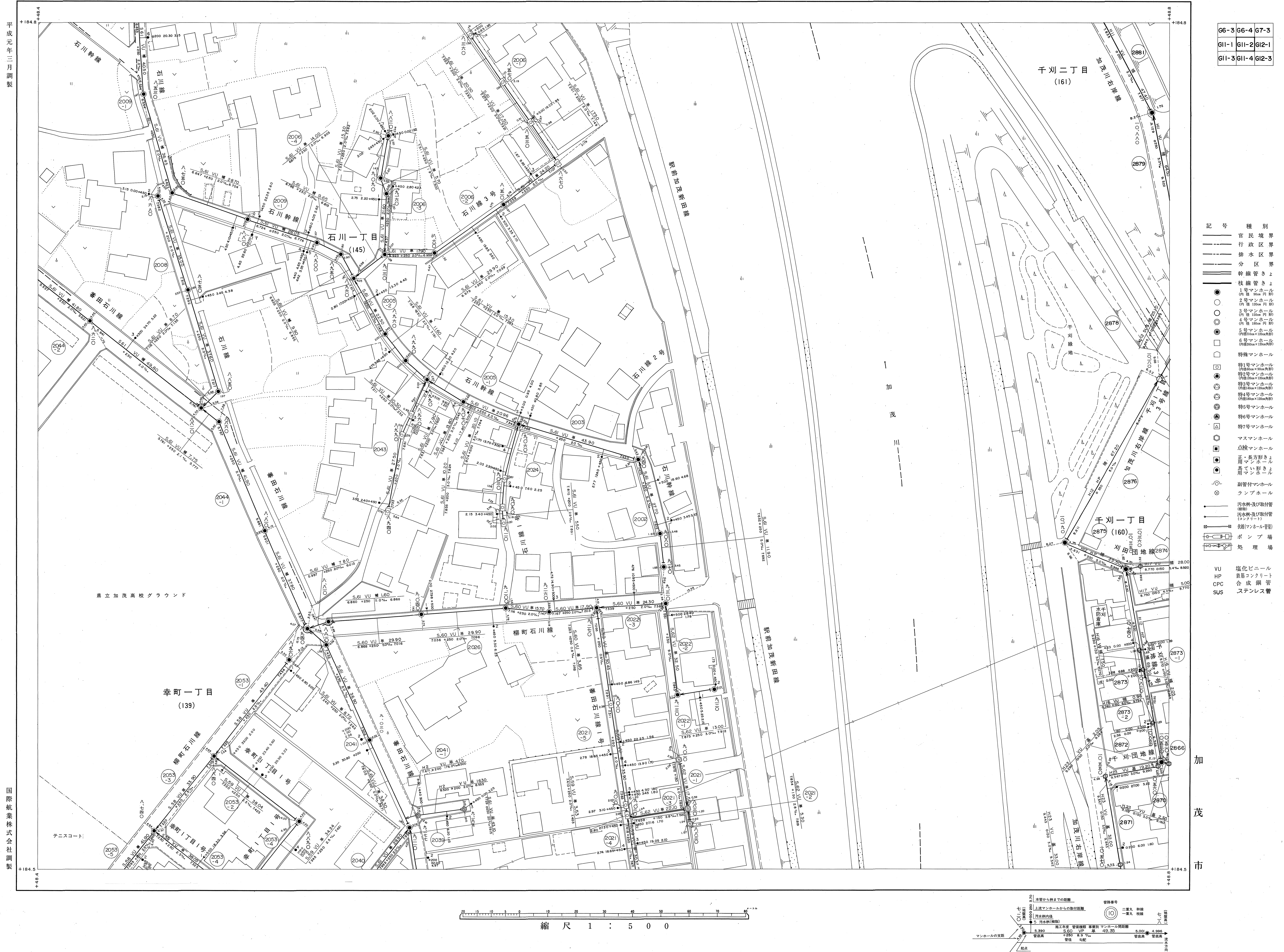
加茂市公共下水道台帳施設平面図 G11-2 (汚水)
